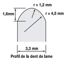
Profil de la dent de lame
